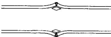
(d) バックリング溶接継手
